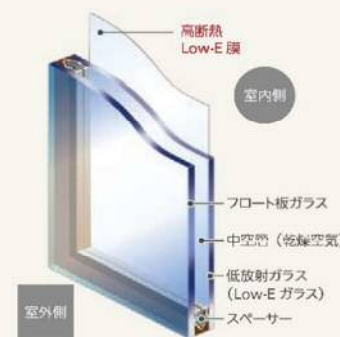
Low-E 二層複層ガラス
