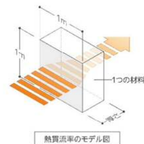
熱貫流率のモデル図
